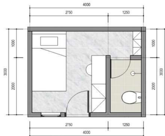
1 KAMAR KOST TYPE 1 (69 KAMAR) - Skala: 1: 50
