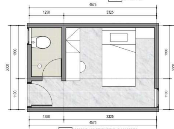
1 KAMAR KOST TYPE 2 (6 KAMAR) - Skala: 1: 50
