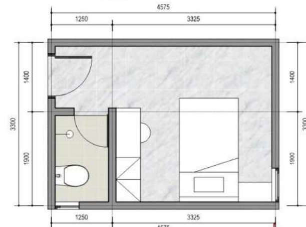
1 KAMAR KOST TYPE 3 (2 KAMAR) - Skala: 1: 50
